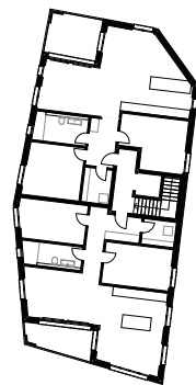
Dachgeschoss
